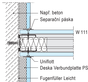
W 631-H1 Napojení na stěnu ze stojek
