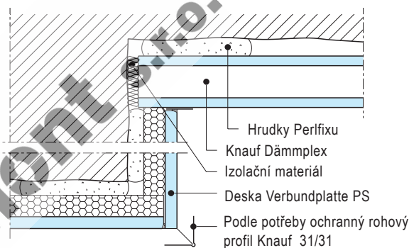
W634-H2 Horizontální řez
