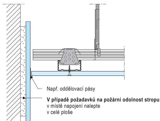
W 611-VO3 Napojenı́ deskového stropu
