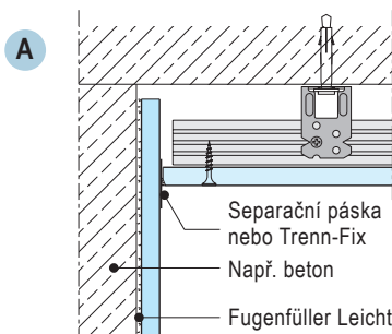
W 611-VO1 Napojenı́ na strop
