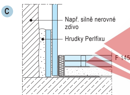
W 611-VU1 Napojenı́ na podlahu
