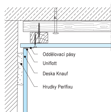
W 611-VO2 Napojenı́ na obklad stropu
