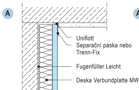
W 624-VO1 Napojenı́ na strop
