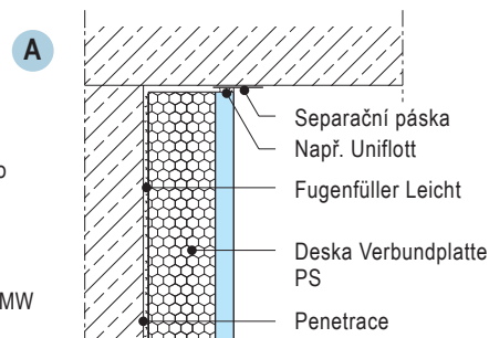
W 631-VO1 Napojenı́ na strop
