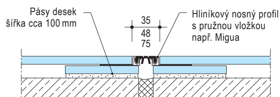
W 611-H3 Dilatační spára s hliníkovým profilem
